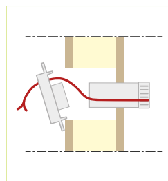
Fig. 8 Fastsättning av suguttag
