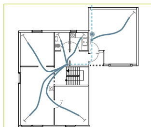
Fig. 2 Placering av suguttag
