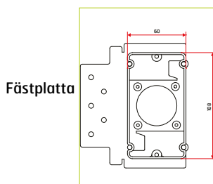
Fig. 7 Montering i befintliga väggar och golv
